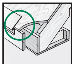
Figure 10 Drip Edge
